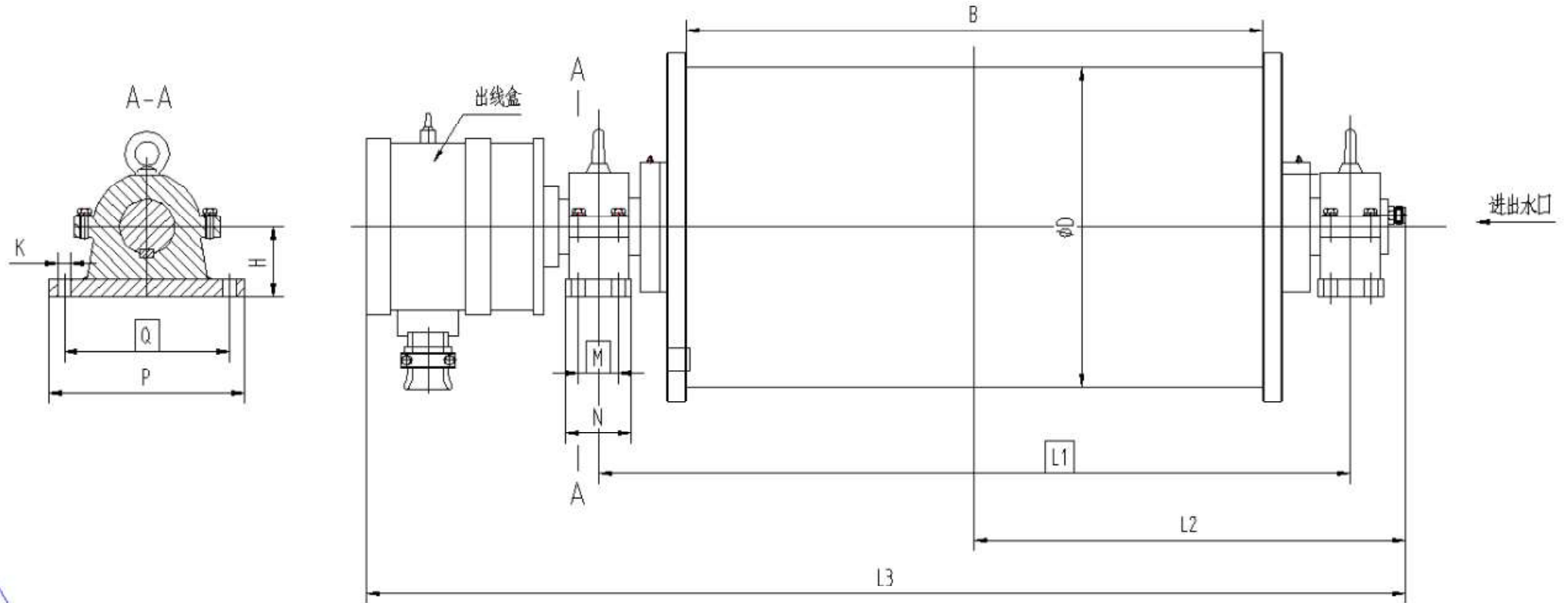
外形图
