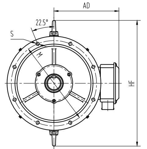
机座号225~280
