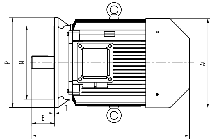
机座号132~280
