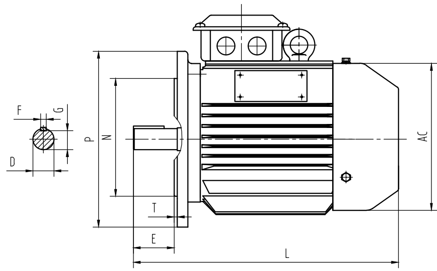
机座号90~112
