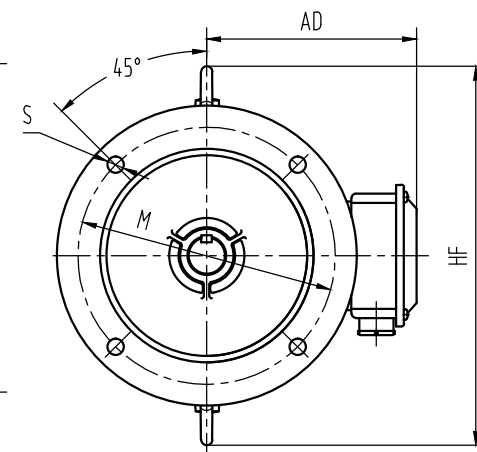
机座号132~200
